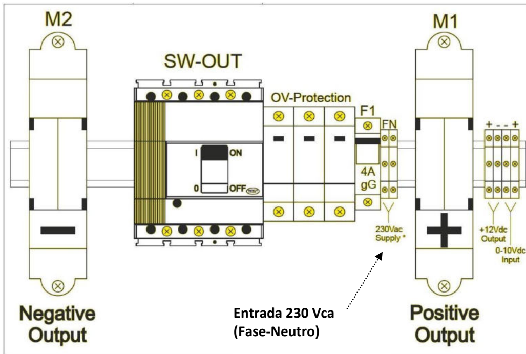
Bornes para la conexión de la tensión de alimentación auxiliar 230 Vca
