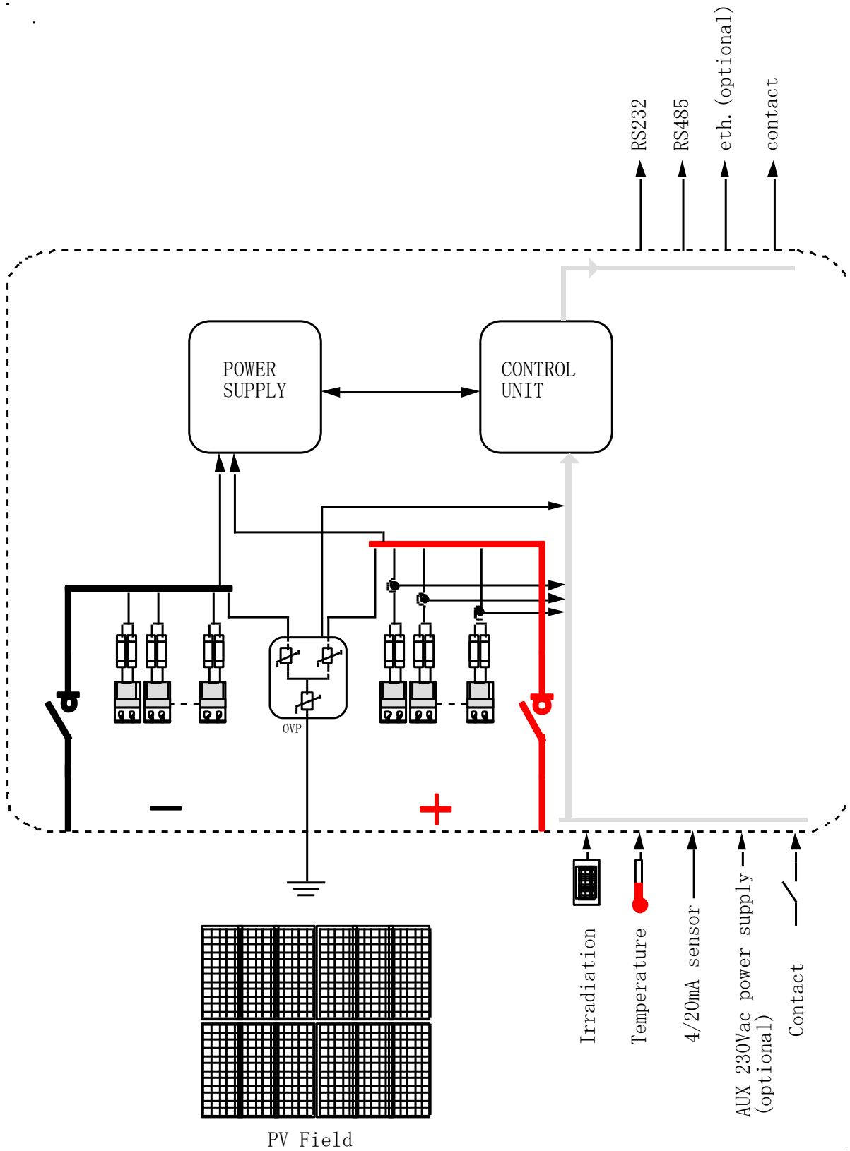
ESQUEMA GENERAL DEL STRING BOX Y PRINCIPALES CONEXIONES DISPONIBLES
